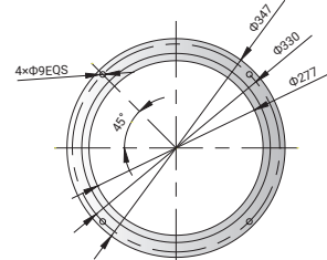
SHR-36U~96U Basisflansch
