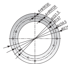
SHR-6U~24U Basisflansch
